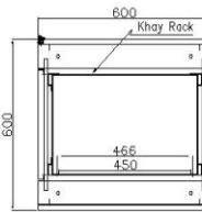
Mặt cắt 1-1
