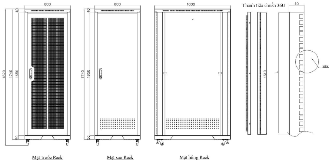
Mặt trước Rack
