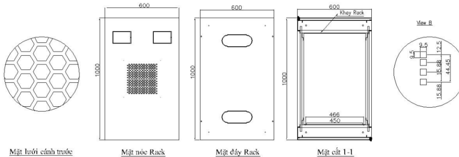
Mặt lưới cánh trước
