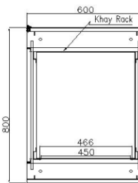
Mặt cắt 1-1
