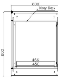
Mặt cắt 1-1
